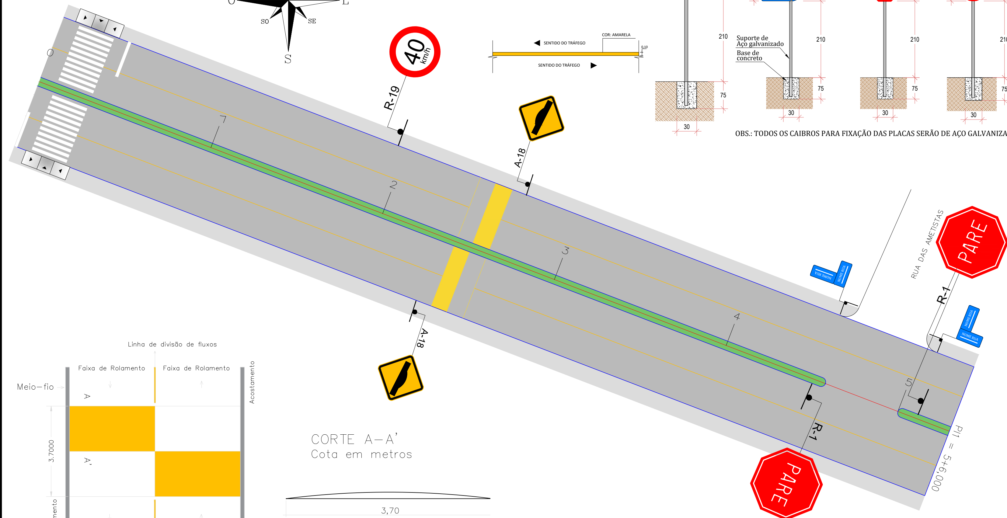
DETALHE LFO-01
