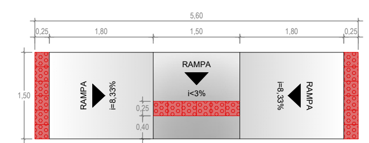
DETALHE DA RAMPA DE ACESSIBILIDADE
