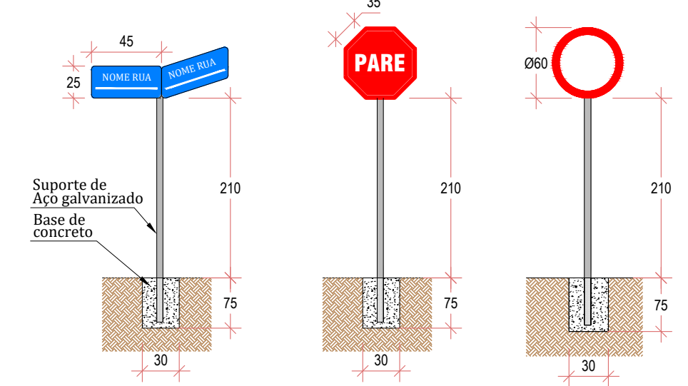
DETALHES CONSTRUTIVOS SINALIZAÇÃO VERTICAL
