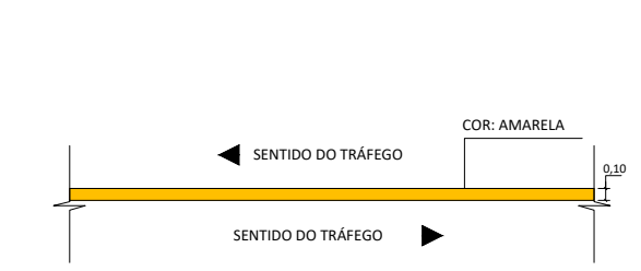
DETALHE LFO-01
