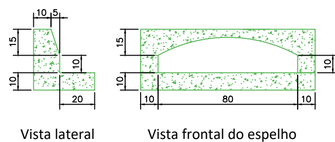
MEIO-FIO TIPO BOCA DE LOBO
